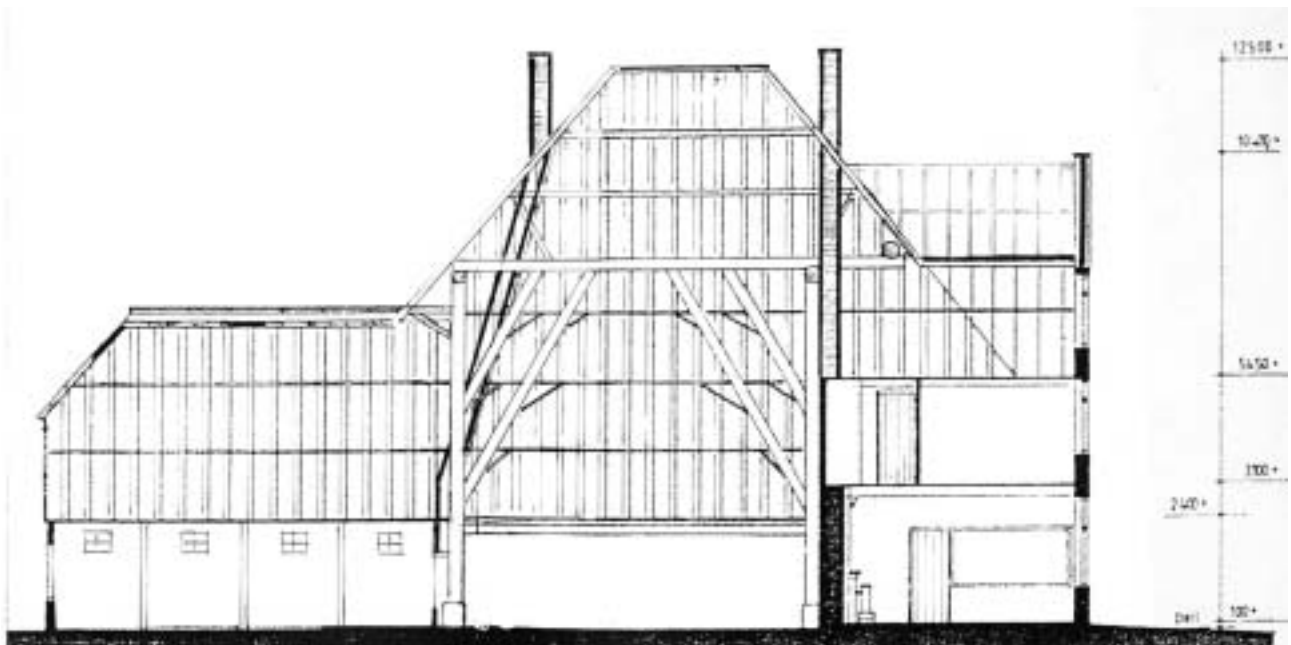
Doorsnede.
